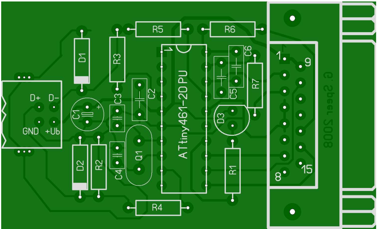
Bestückungsseite
